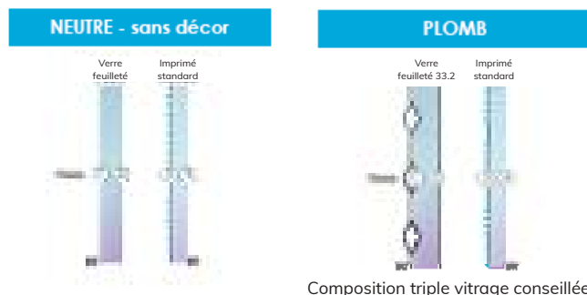
Composition triple vitrage conseillée
